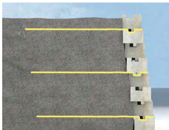
شکل ۲۲-۱۸ بلوک بتنی مدولار با کلید برشی
