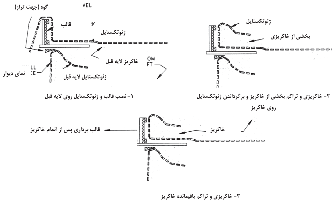
شکل ۲۲-۲۱ مراحل اجرای دیوار خاک مسلح بدون نما
