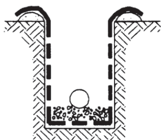
۳- اجرای مصالح زیرین و نصب لوله
