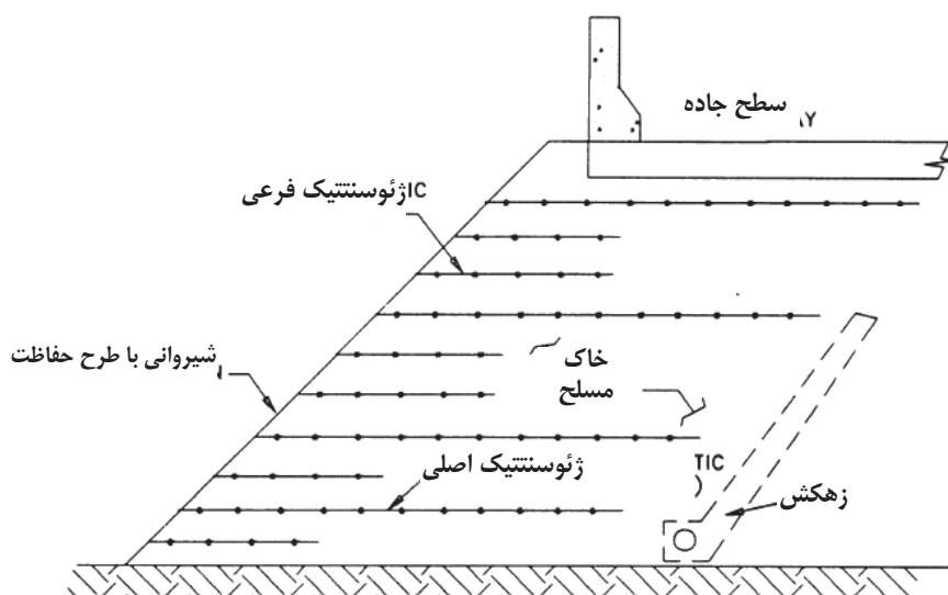
شکل ۲۲-۱۳ شیب خاکی مسلح
