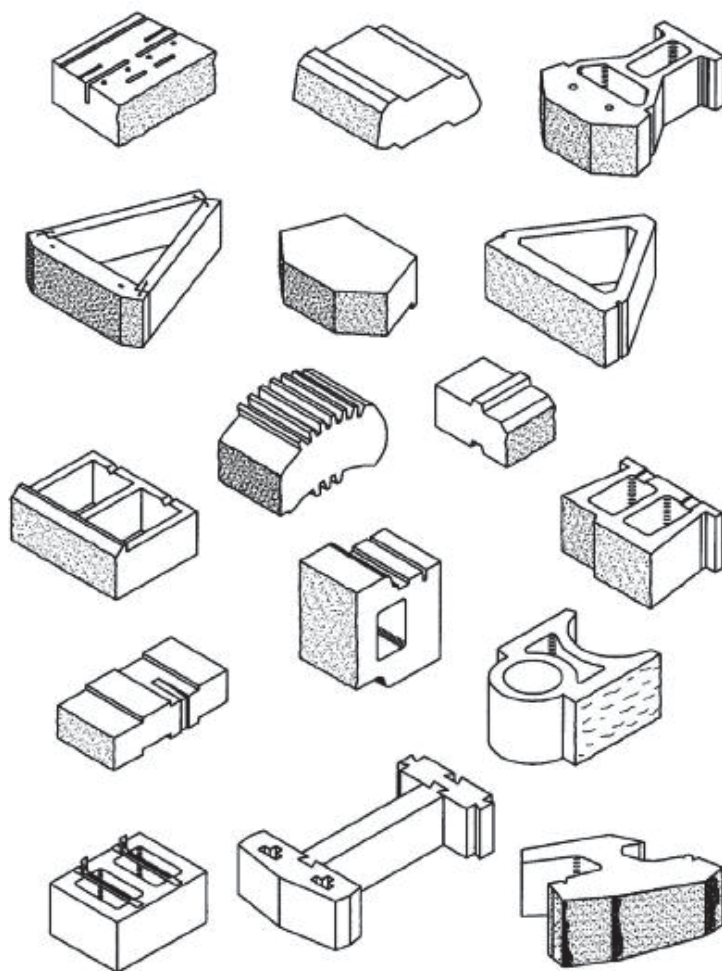
شکل ۲۲-۱۹ برخی از انواع قطعات بتنی مدولار
