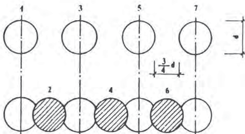
شکل ۶-۳ فاصله بین شمع‌ها، 0.75d قطر شمع‌ها
