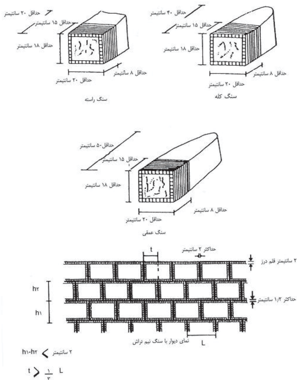
شکل ۵-۶ بنایی با سنگ نیم سرتراش Moellon Pique
