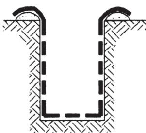
۲- نصب ژئوتکستایل
