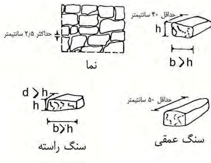
شکل ۱-۵ بنایی با سنگ قواره Uncoursed Rubble Masonry (UR) Moellon Brut
