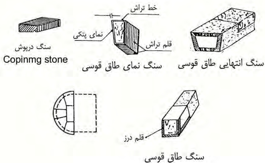
شکل ۲-۵ بنایی با سنگ تمام تراش Fine Ashlar Masonry (FA) Moellon Dappareil
