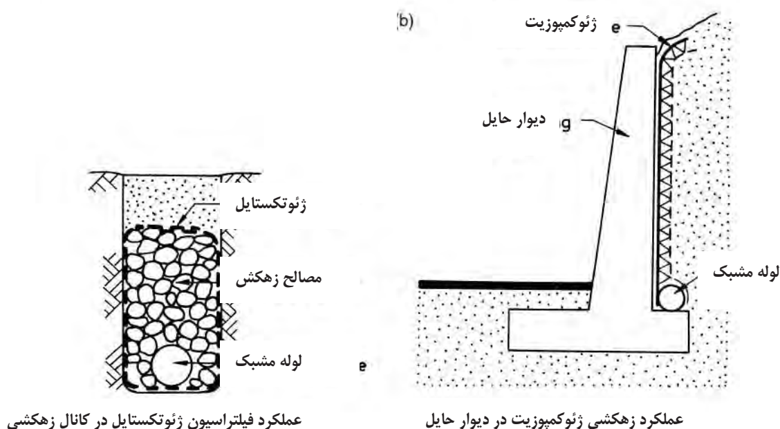
شکل ۲۲-۶ نمونه‌ای از عملکرد فیلتراسیون و زهکشی ژئوسنتتیک‌ها
