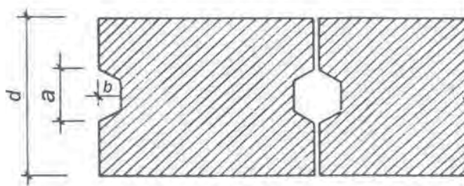
شکل ۶-۱ سپرهای بتن فولادی
