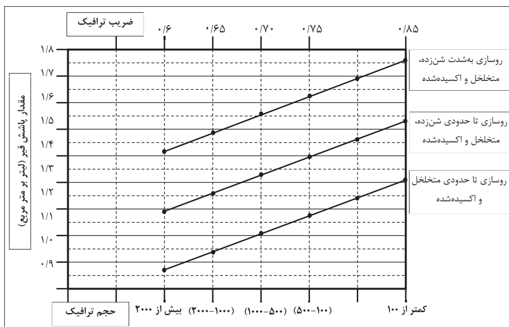
شکل ۲-۱۷ نمونه‌ای از نمودار تعدیل مقدار قیر برای زمان اجرای آسفالت سطحی
