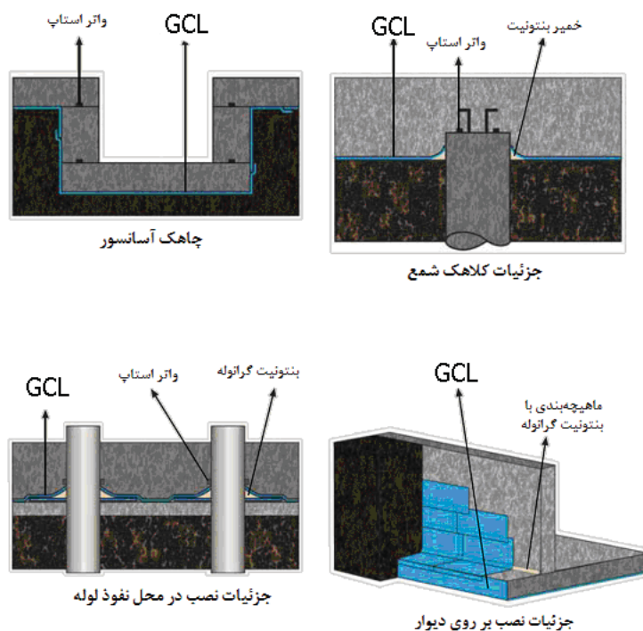
شکل ۲۲-۲۶ نحوه اجرای جی سی ال در اطراف سر شمع و دیواره گود و محل اتصال
