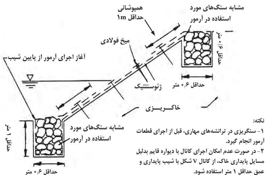
شکل ۲۲-۹ سیستم کنترل فرسایش با ترانشه‌های مهاری
