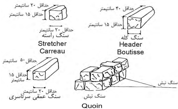
شکل ۴-۵ سنگ عمقی سرتاسری Through Stone Parpaing
