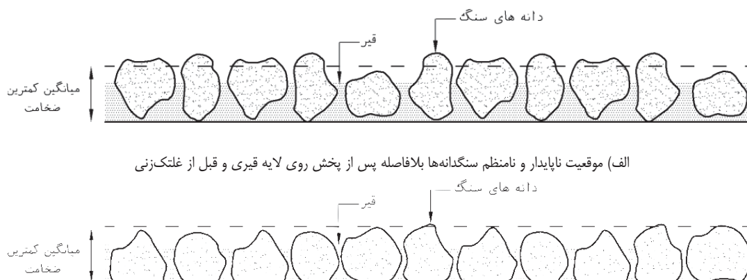
ب) موقعیت پایدار و تثبیت‌شده سنگدانه‌ها پس از بهره‌برداری نسبتاً طولانی‌مدت که روی جبهه‌های پهن خود در لایه قیری فرو نشسته‌اند
