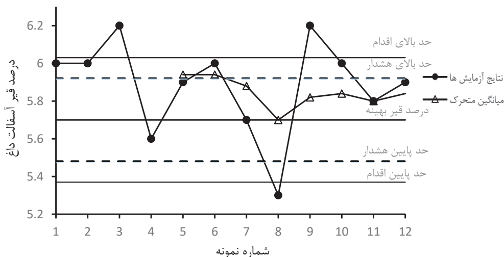
شکل ۲۰-۴- نمودار کنترلی درصد قیر آسفالت داغ
