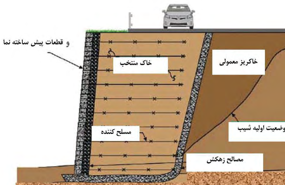
ب) مسطح کننده ژئوگریدی با نمای بلوک مدولار بتنی
