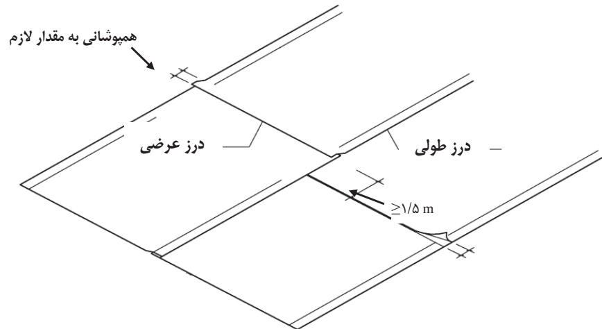
شکل ۲۲-۳ حداقل فاصله افقی درزهای عرضی نسبت به هم
