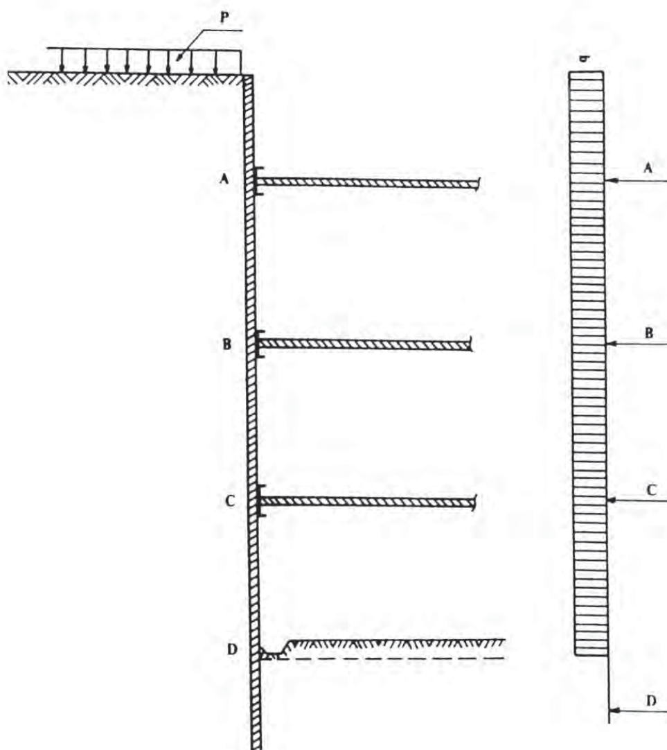
شکل ۶-۶ سیستم استاتیکی یک سیپر برای مراحل مختلف گودبرداری
