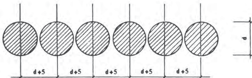
شکل ۶-۲ یک سری شمع در کنار یکدیگر
