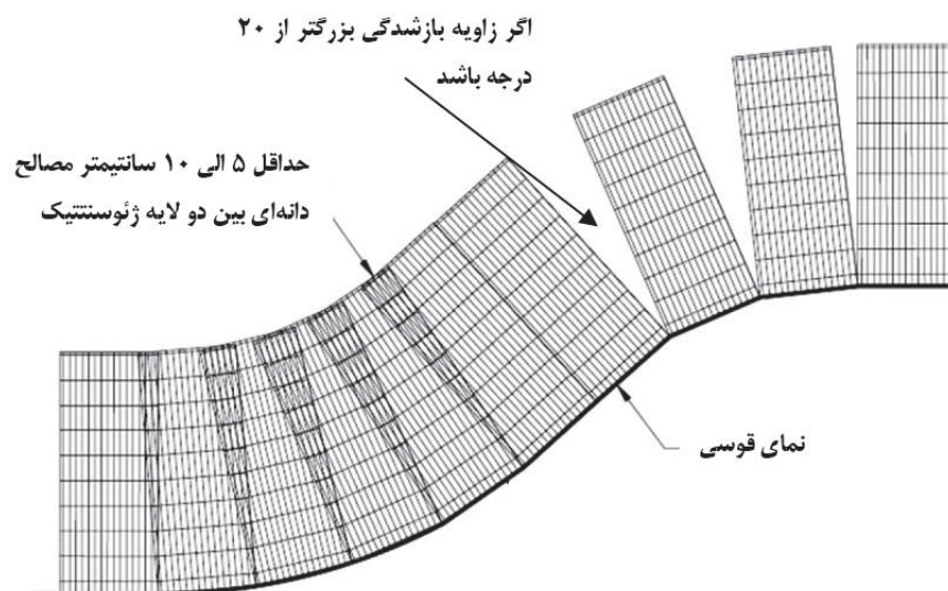
شکل ۲۰-۲۲ نمونه‌ای از نصب ژئوسنتتیک در دیوار با نمای قوسی
