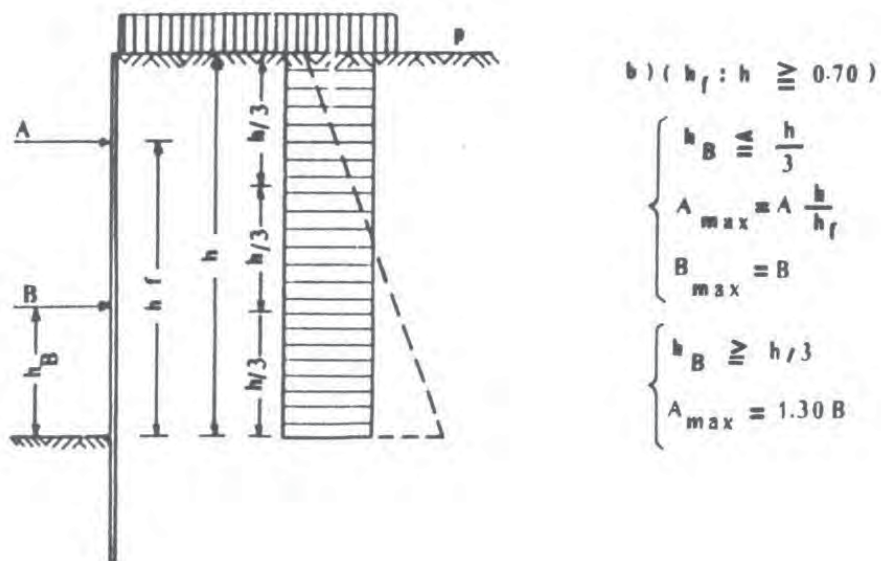
شکل ۶-۸ سپر دارای دو تکیه‌گاه یا دو مهار
