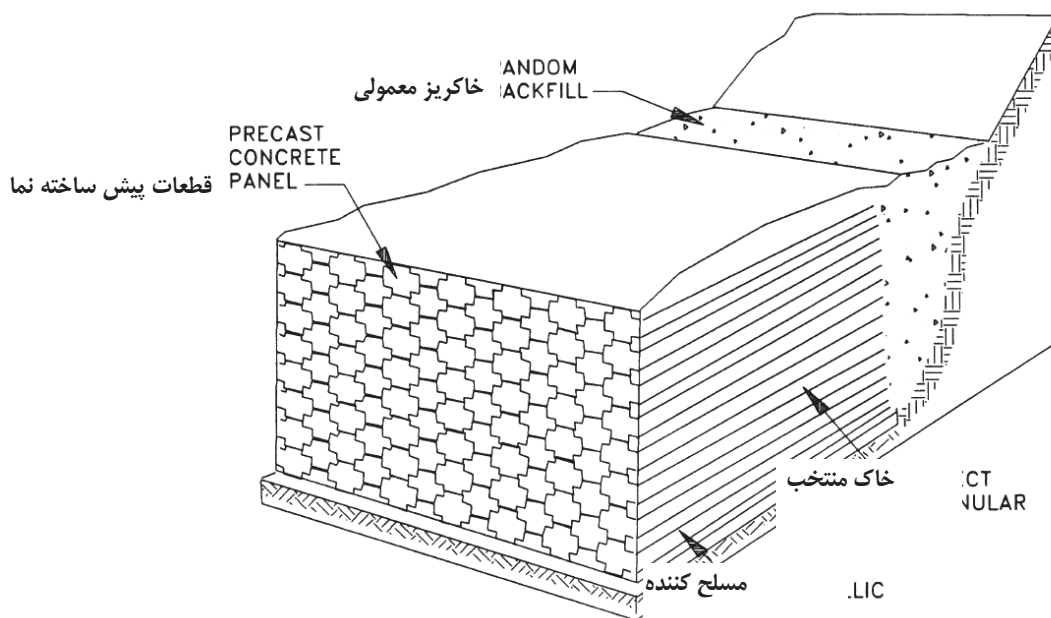
الف) مسطح کننده تسمه فلزی با نمای پانلی
