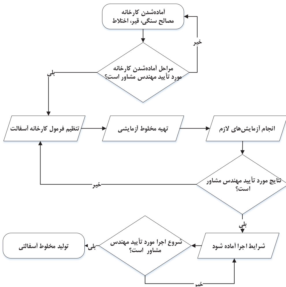
شکل ۲۰-۱- چرخه تولید آسفالت آزمایشی
