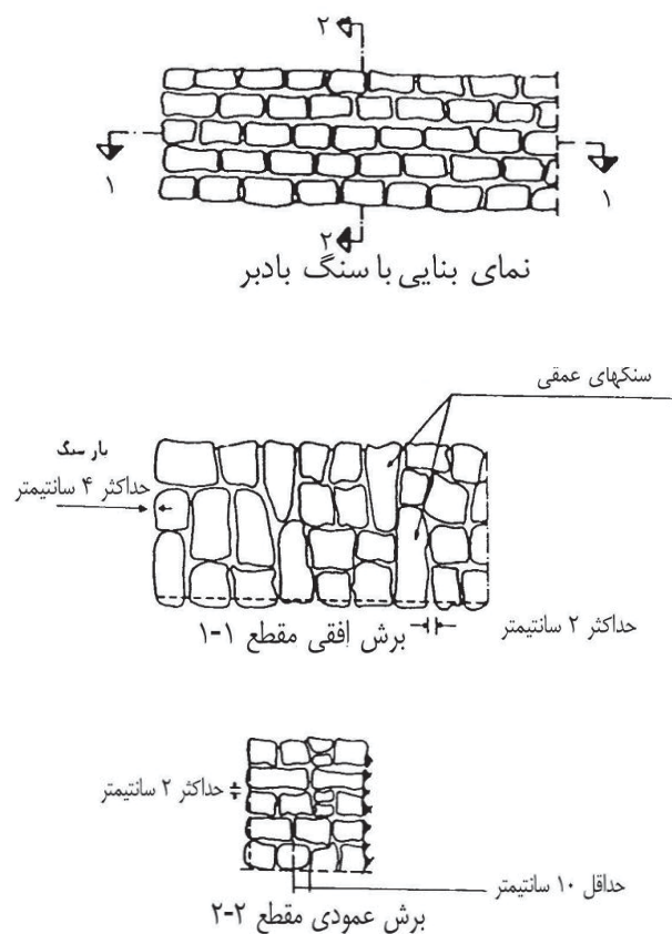
شکل ۳-۵ بنایی با سنگ بادبر Coursed Rubble Masonry
