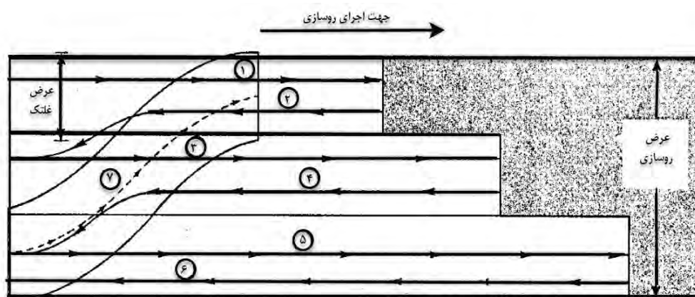
شکل ۲-۲۰ نمونه پیشنهادی از الگوی غلتک‌زنی با استفاده از غلتک فولادی استاتیکی
