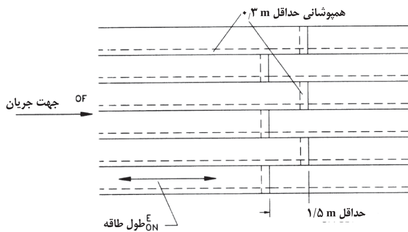
الف - نما
