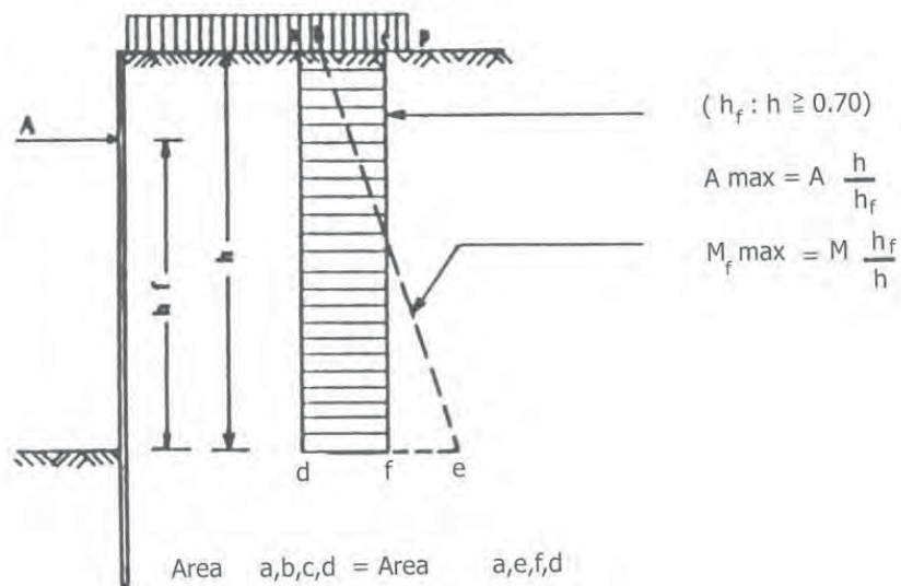
شکل ۶-۷ سپر دارای یک تکیه‌گاه یا یک مهار
