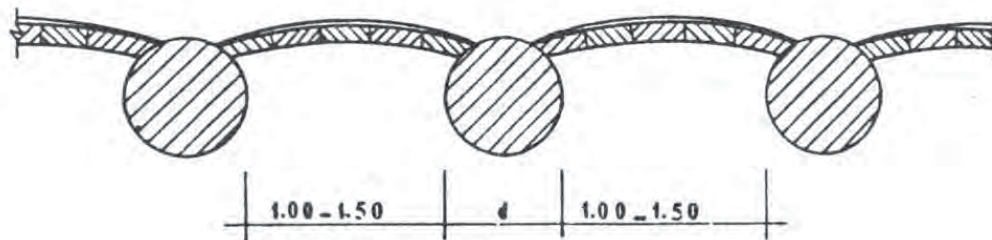
شکل ۶-۴ شمع‌ها به فاصله یک متر الی ۱/۵ متر از یکدیگر
