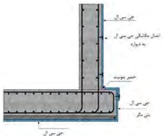
شکل ۲۲-۲۴- اجرای جی سی ال در اطراف فونداسیون
