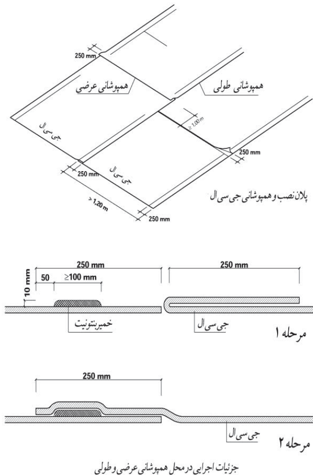
شکل ۲۲-۲۳ اجرای جی سی ال در کف
